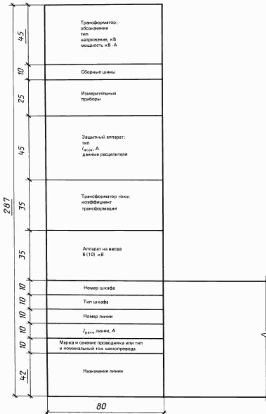
Принципиальная схема КТП
